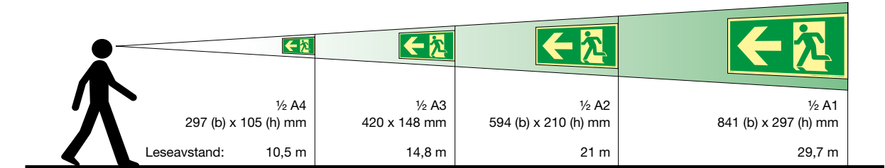
Illustrasjonen viser tabell med leseavstand for etterlysende skilt i rømningsveien.
